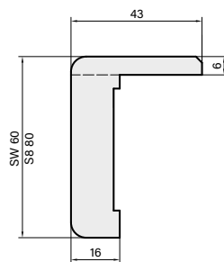
Rohový prvok zárubne SW, S8 obložka standard
