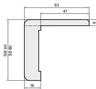
Rohový prvok zárubne SW, S8 predĺžená obložka o 2 cm
